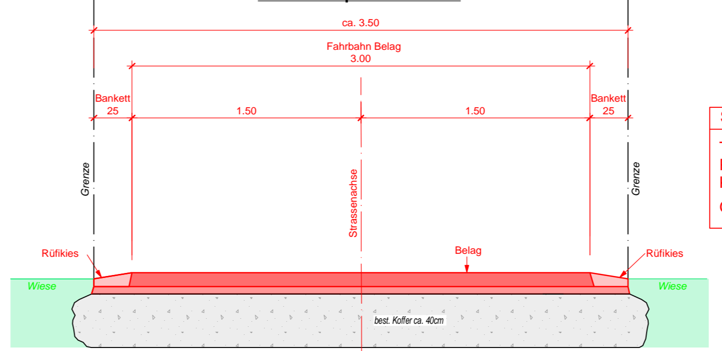
Normalprofil 1:25
