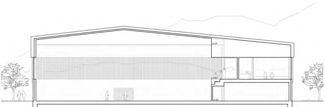
Schnitt Mehrzweckhalle-Tribüne-Garderoben
